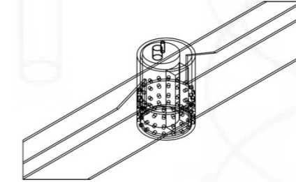
Système de pompage d'eau de surface
