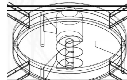
Support mélangeur de surface
